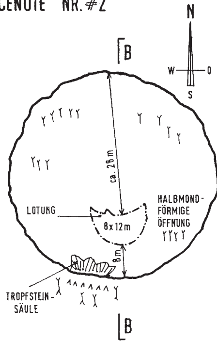
GRUNDRISS
