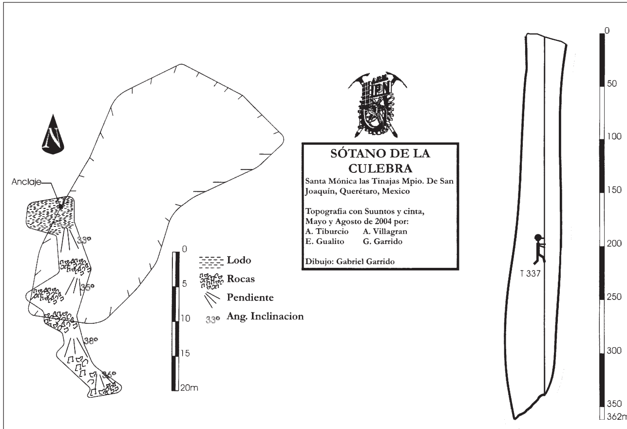
Sótano de la Culebra Santa Mónica las Tinajas, Mpo. San Joaquín Querétaro AMCS Activities Newsletter 28, p. 10, 2005
