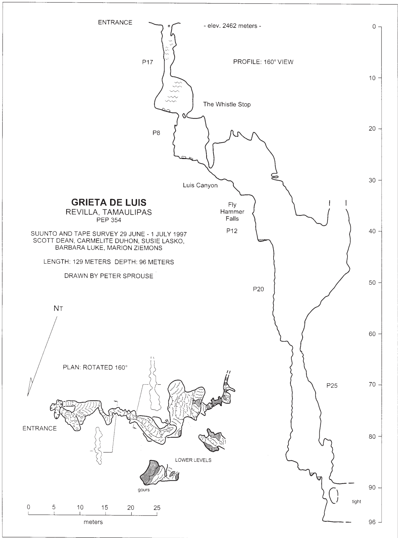
Grieta de Luis Revilla, Mpo. Güémez Tamaulipas Death Coral Caver, no. 7, p. 16, 1997
