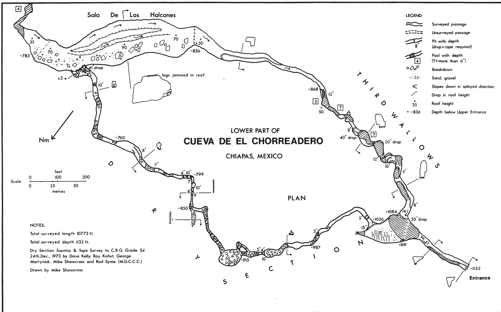
Cueva de el Chorreadero (part) Mpo. Chiapa de Corzo Chiapas Canadian Caver, v. 6, no. 1, p. 62, 1974
