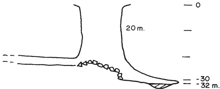
SOTANO del LLANO SIN NOMBRE memory sketch by C. Yonge
