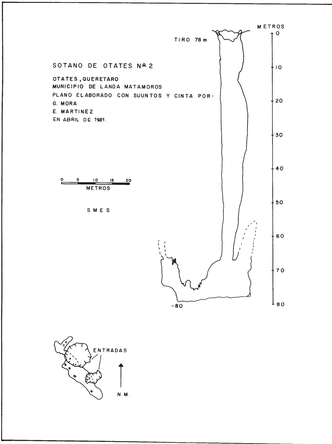
Sótano de Otates no. 2 Otates, Mpo. Landa de Matamoros Querétaro
