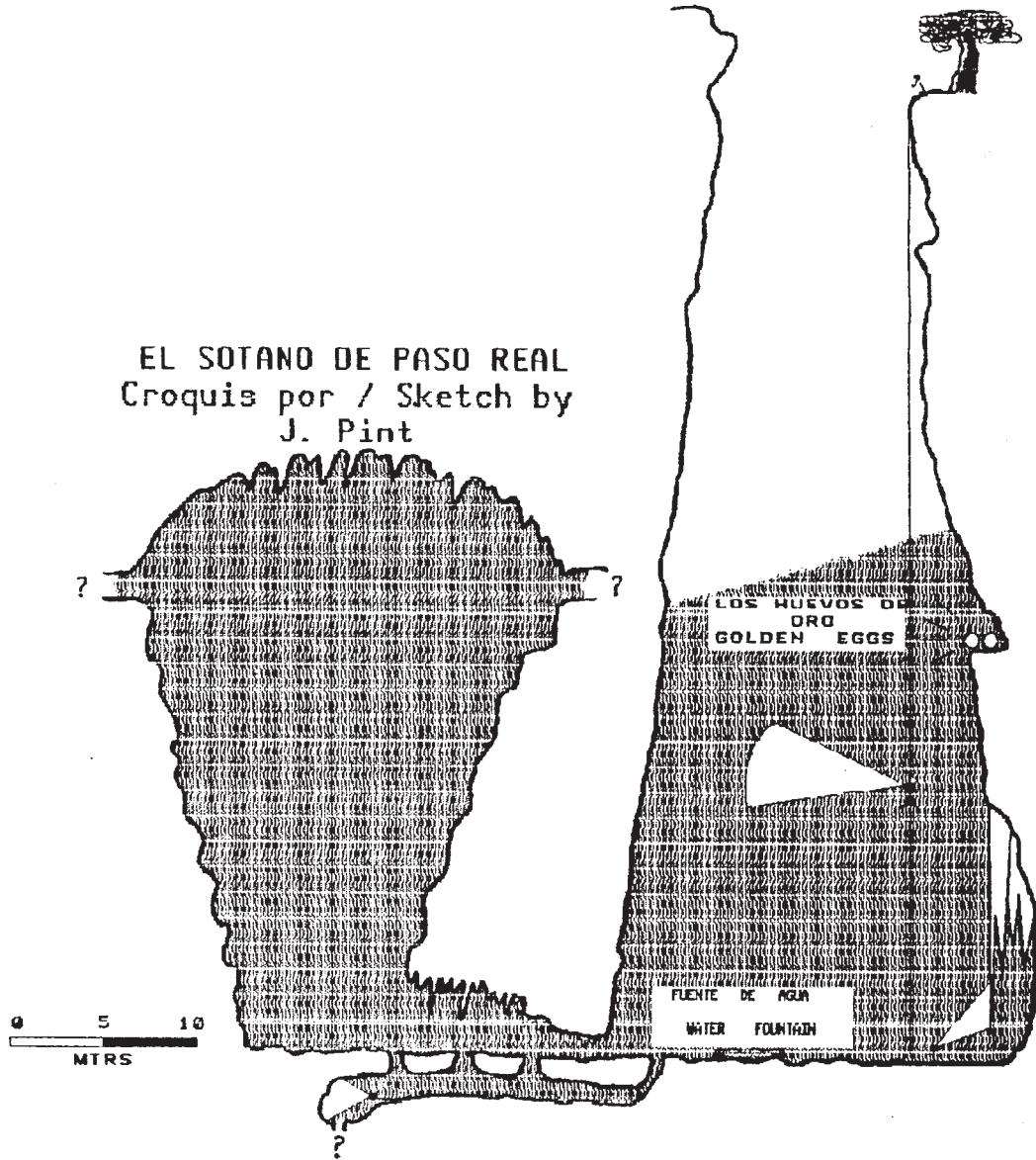
Sótano de Paso Real Paso Real, Mpo. San Miguel Jalisco Subterráneo, no. 7, p. 11, 1991
