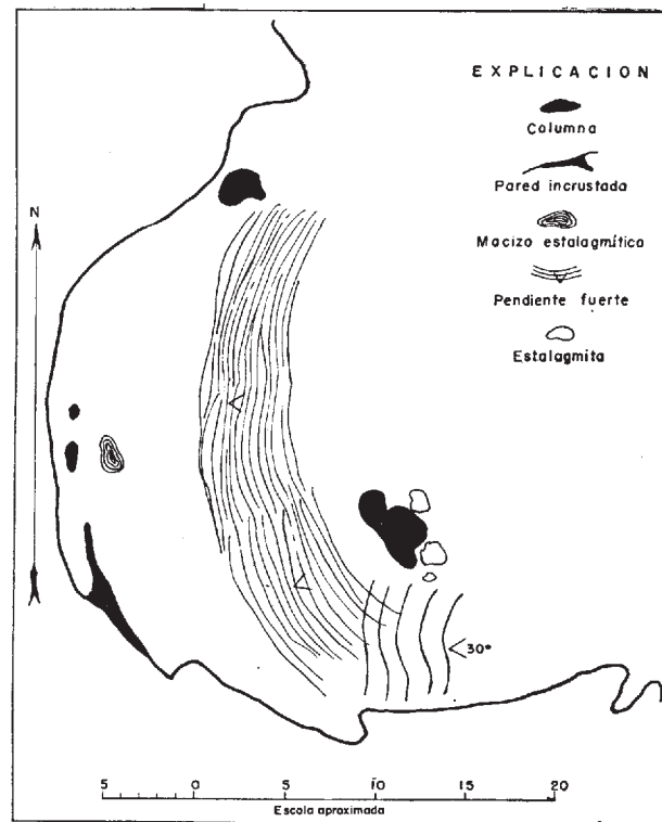
Fig. 3 CUEVA DEL TAPATÍO, XILITLA, S. L. P. Plano esquemático
