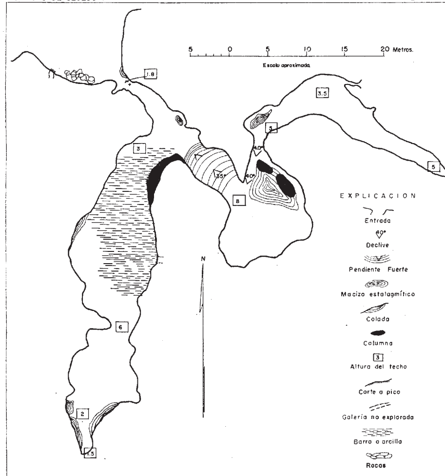
CUEVA DE LOS CUCHOS, XILITLA, S.L.P. Plano esquemático
