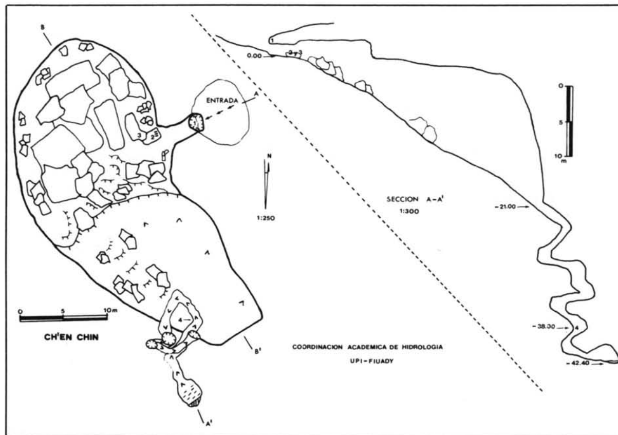
Figura 5. Plano de Aktun Ch'en Chin , Planta y Sección. 1: Caras grabadas en la entrada. 2: Paneles I y II. 3: Panel III. 4: Paneles IV y V.
