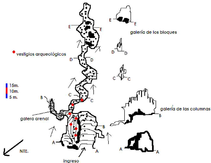
Topografía cueva del Guayabo2, planta, Topografía por: Gabriel Merino.
