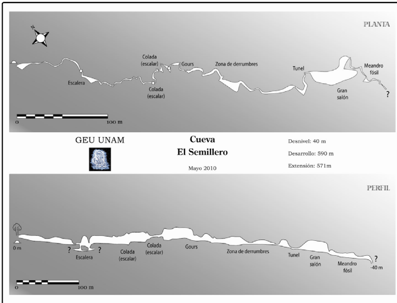
Cueva el Semillero Zongolica Veracruz Mundos Subterráneos 21, p. 71, 2010
